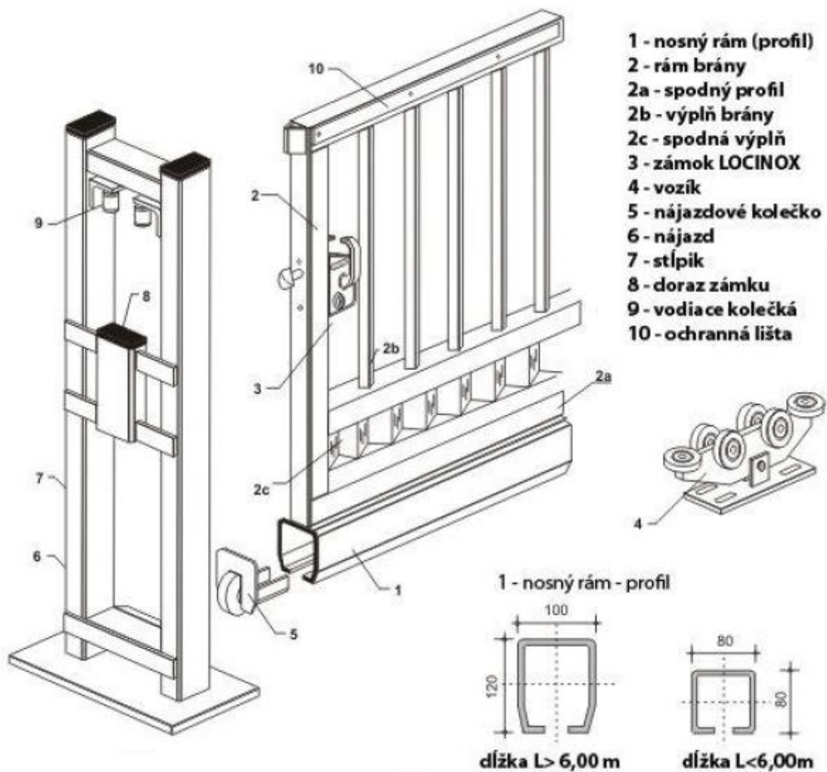
Detail - brána samonosna, typ BST
